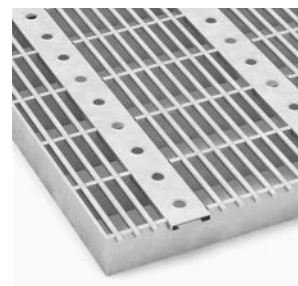
AR1-25 raapelista Silmäkoko: k/k 60x10 mm
