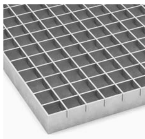
A22X22 Silmäkoko: k/k 22x22 mm
