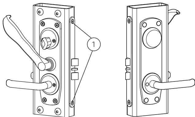
ASSA 722-50 + ASSA 179A
