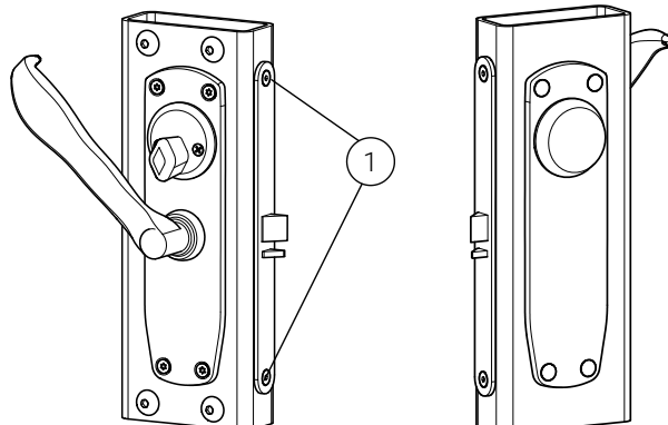
ASSA 732-50 + ASSA 179B
